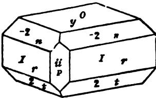
Lederite.
